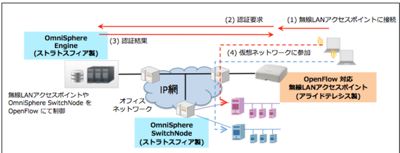
図 1: OmniSphere と無線 LAN アクセスポイントの構成図
