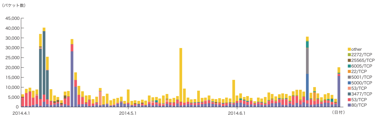
図-4 DDoS攻撃によるbackscatter観測(観測パケット数、ポート別推移)
