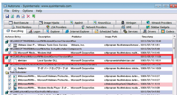
図-13 vawtrakによって改変されたレジストリ
