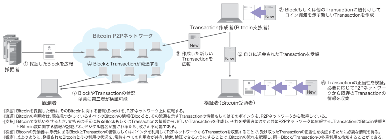
図-19 Bitcoinの仕組み
