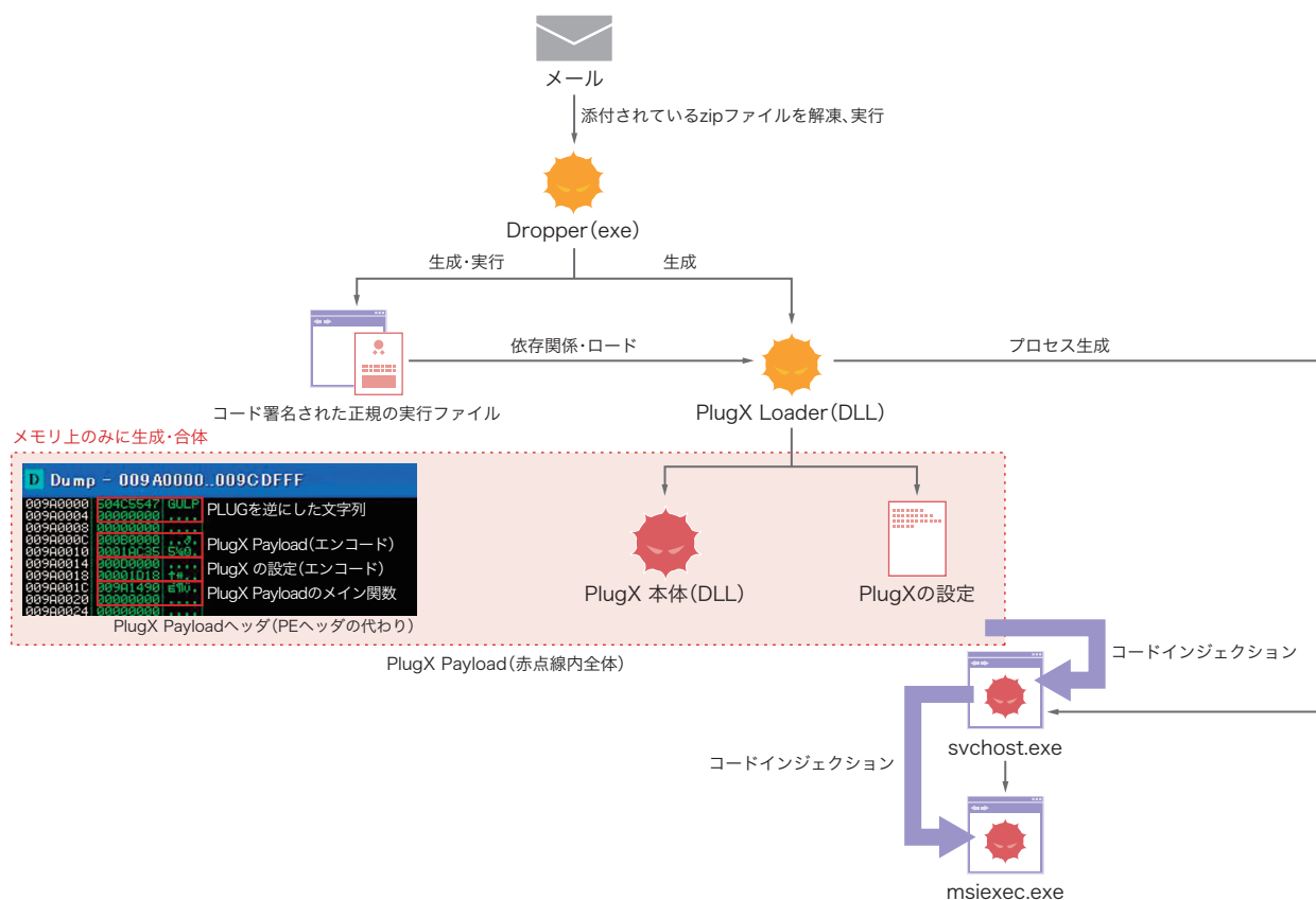
図-13 PlugXの実行フロー
