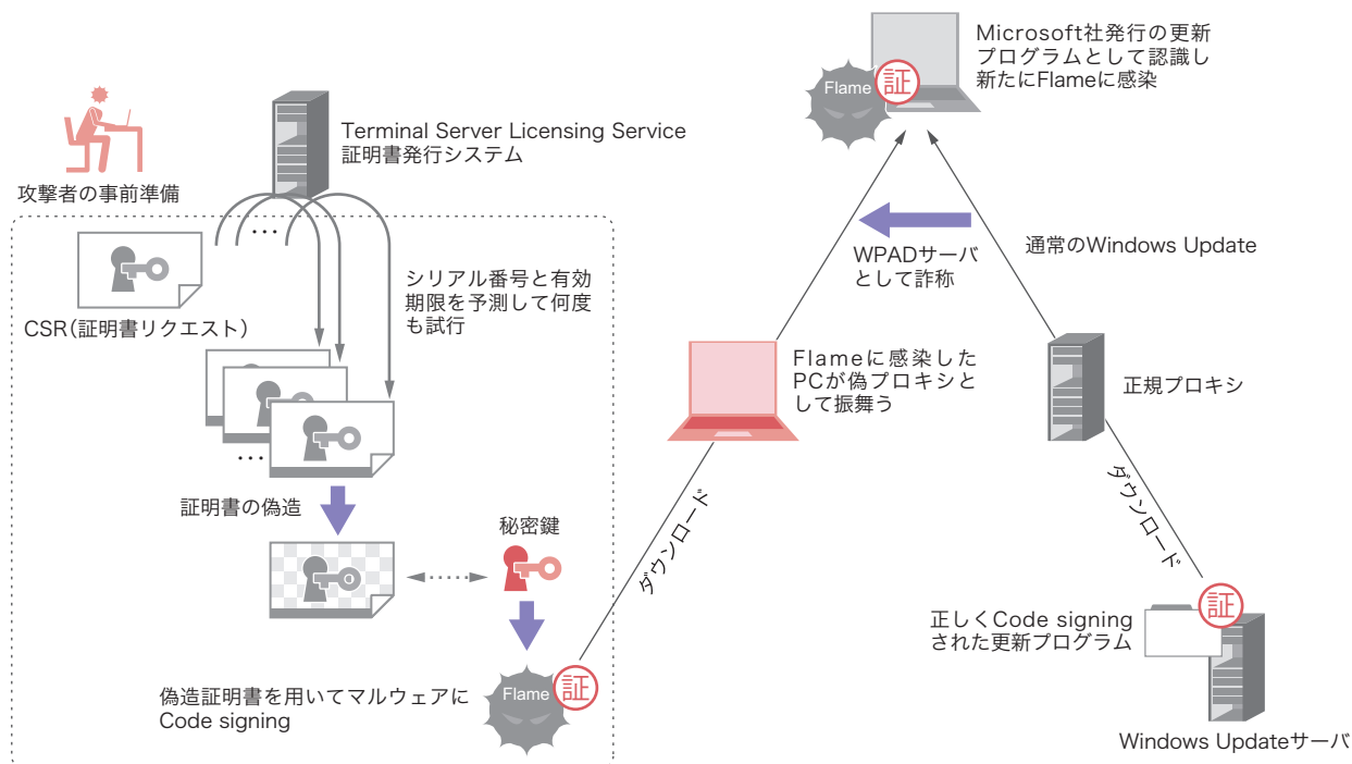
図-12 マルウェアFlameの動作概要
