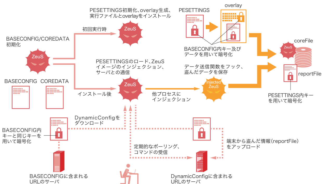
図-13 Zeusボットの感染動作
